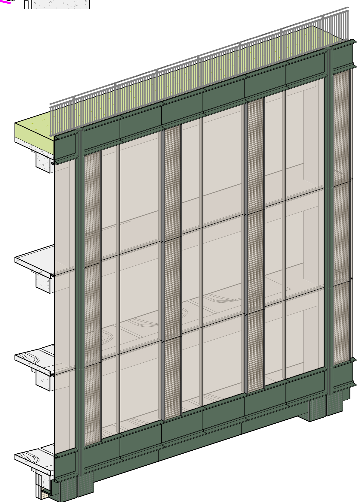
4 AXONOMETRIC 1/2" = 1'-0"
